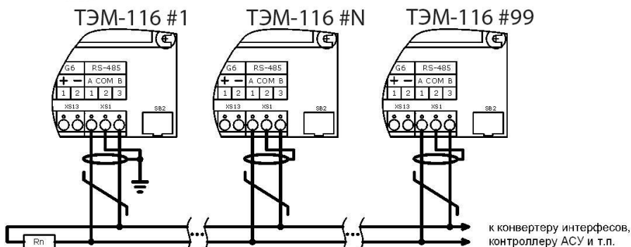
Схема электрических соединений при организации сети
