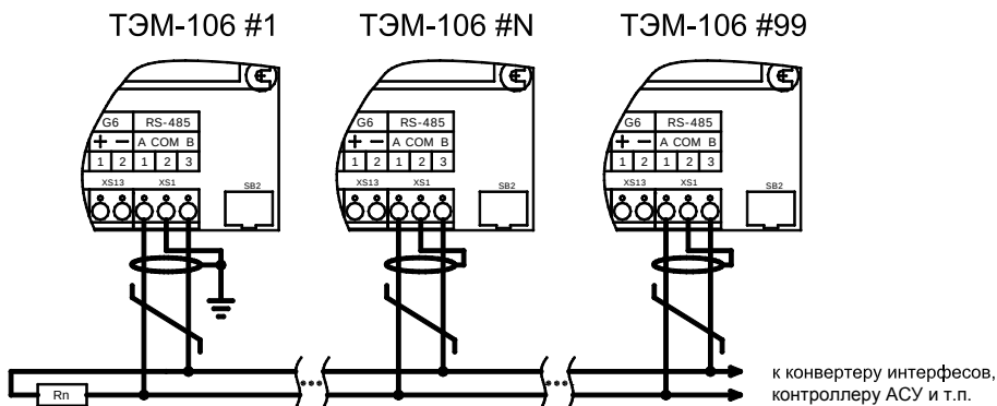
Схема электрических соединений при организации сети
