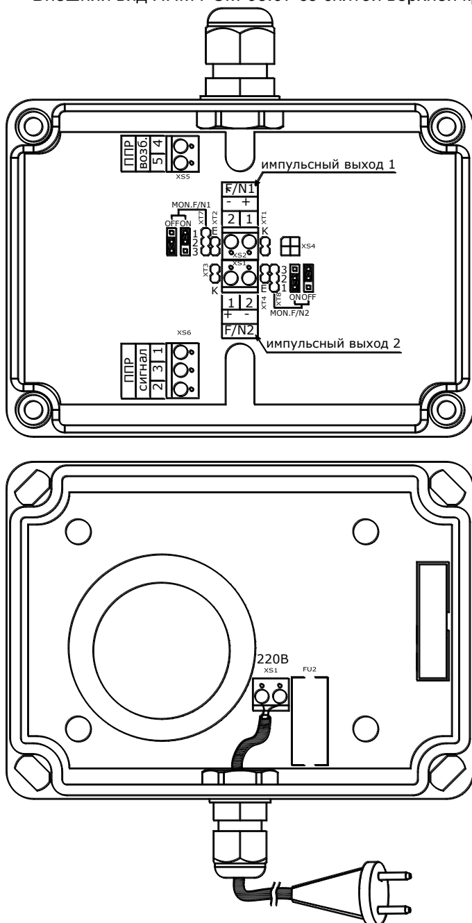
Внешний вид ППМ РСМ-05.07 со снятой верхней крышкой
